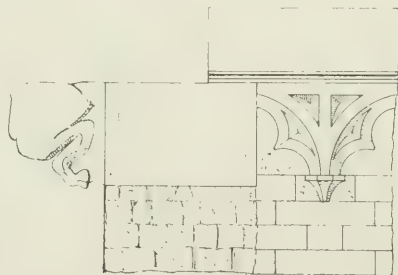
Fig. 66. Fragment balustrady z rynną.
